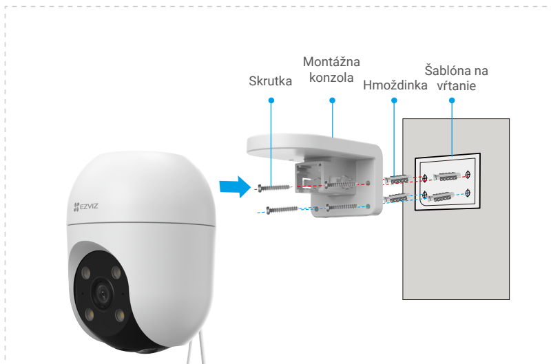
Obr. 2 Nástenné upevnenie
