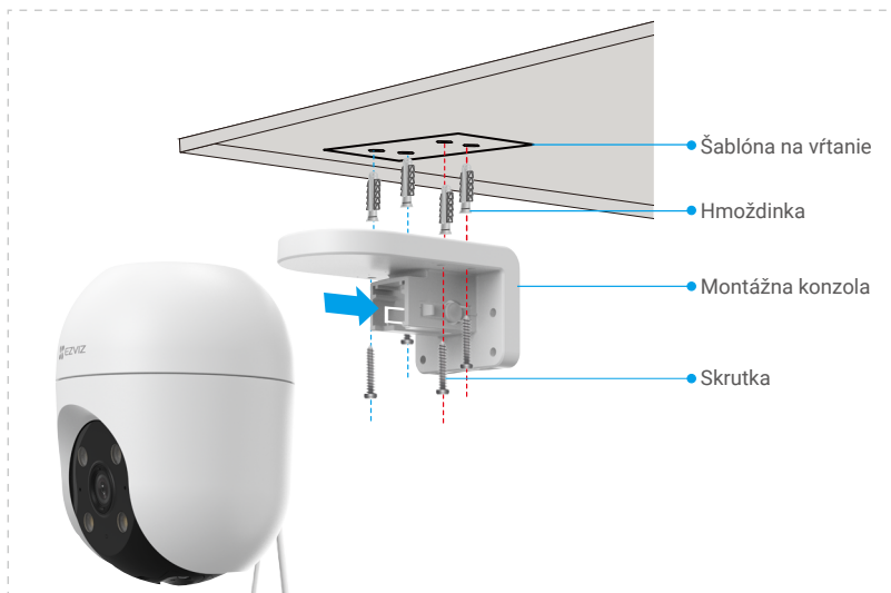
Obr. 1 Stropné upevnenie
